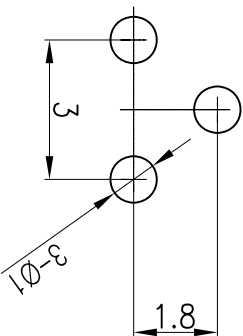
PCB线路板安装图(±0.1)
