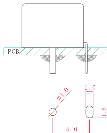
PCB焊锡插脚孔位
