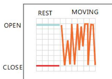
触发波形图
