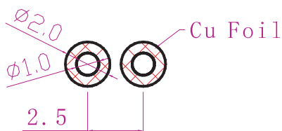
P.C.B. Layout (DIP)
