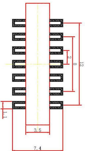
PCB板位置尺寸
