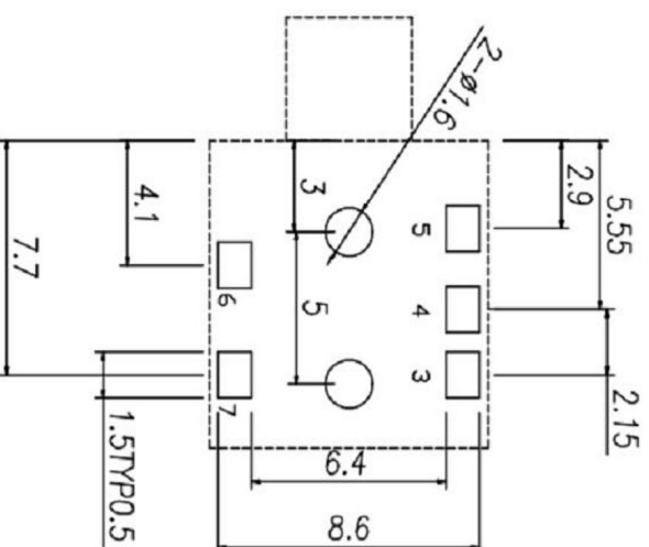
线路板安装尺寸示意图
