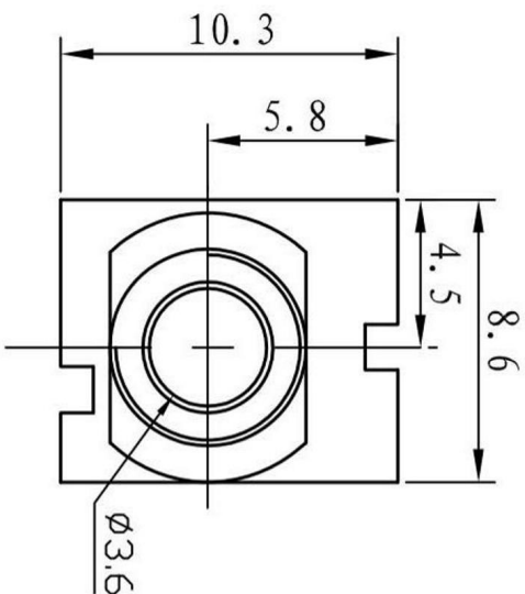
线路板安装尺寸示意图
