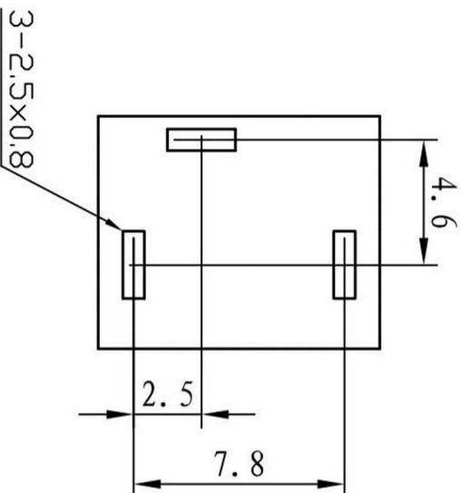
线路板安装尺寸示意图
