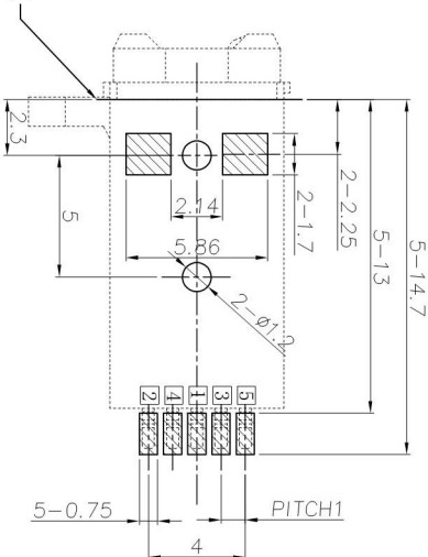
PCB EDGE
