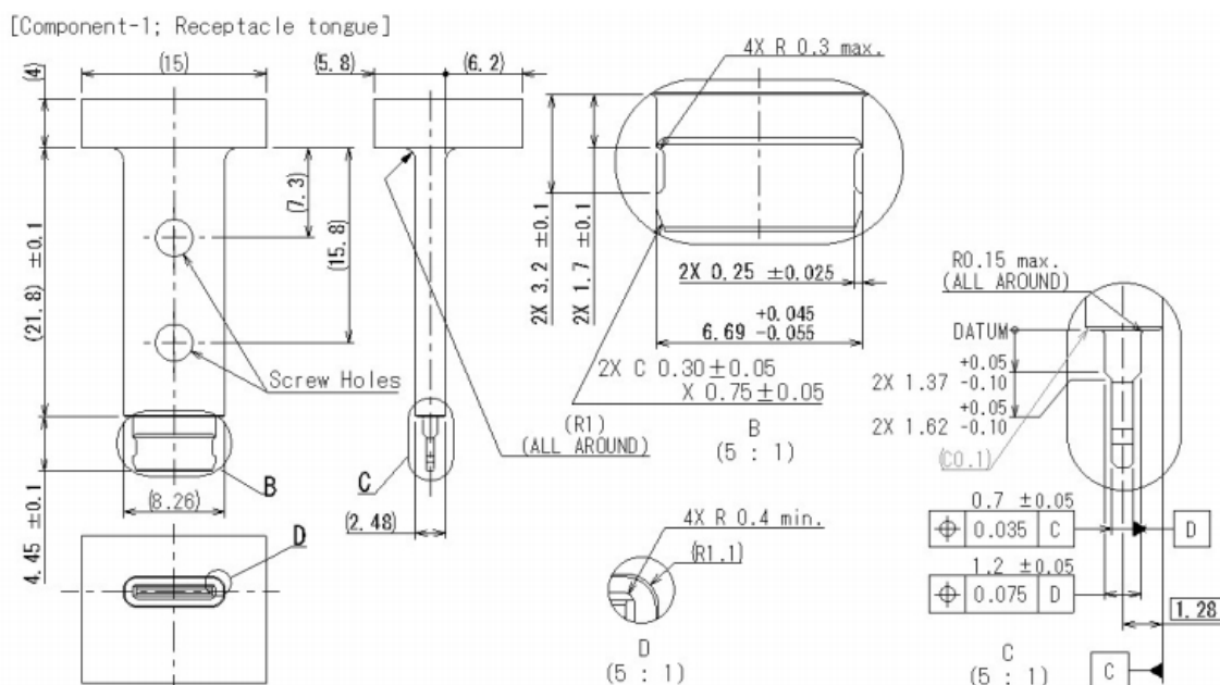
Receptacle tongue
