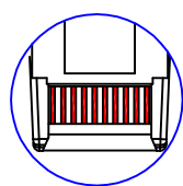
DETAIL C SCALE 2:1 (Switch连接) 母线接头
