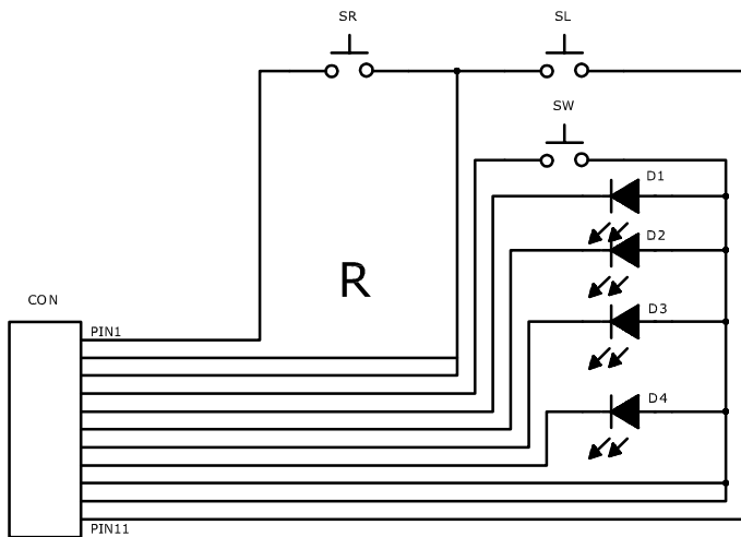
灯板线路图
