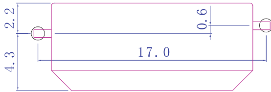
P. C. B. Layout (DIP) 开关放置电路板孔位
