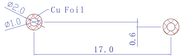
P. C. B. Layout (DIP) 焊盘位
