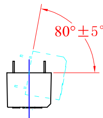
恢复动作角度: 80^{\circ} \pm 5^{\circ}
