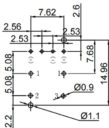
P.C.B . Layout
