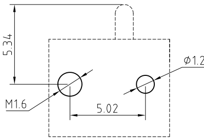
印制电路板及焊接安装孔参考图 (自 A 方向看)
