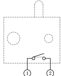
电路图：常开式(N.O) 1个电路1个接点 端子排列（自 A 方向看）
