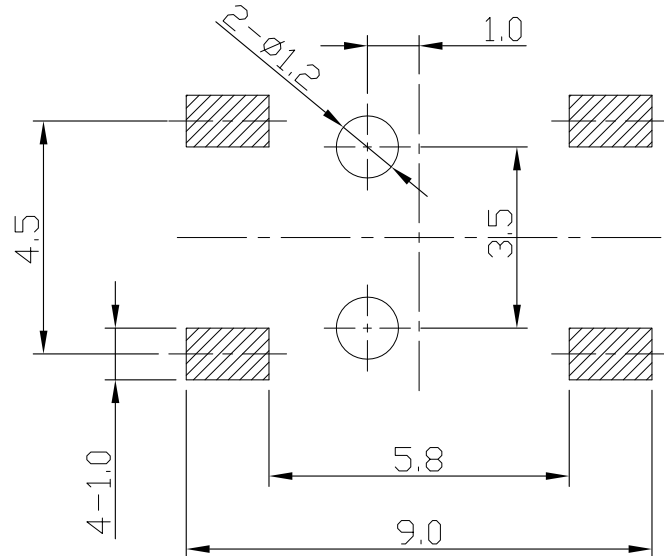
P.C.B LAND DIMENSION
