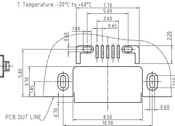
P.C.B LAYOUT
