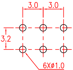
P.C.B. LAYOUT
