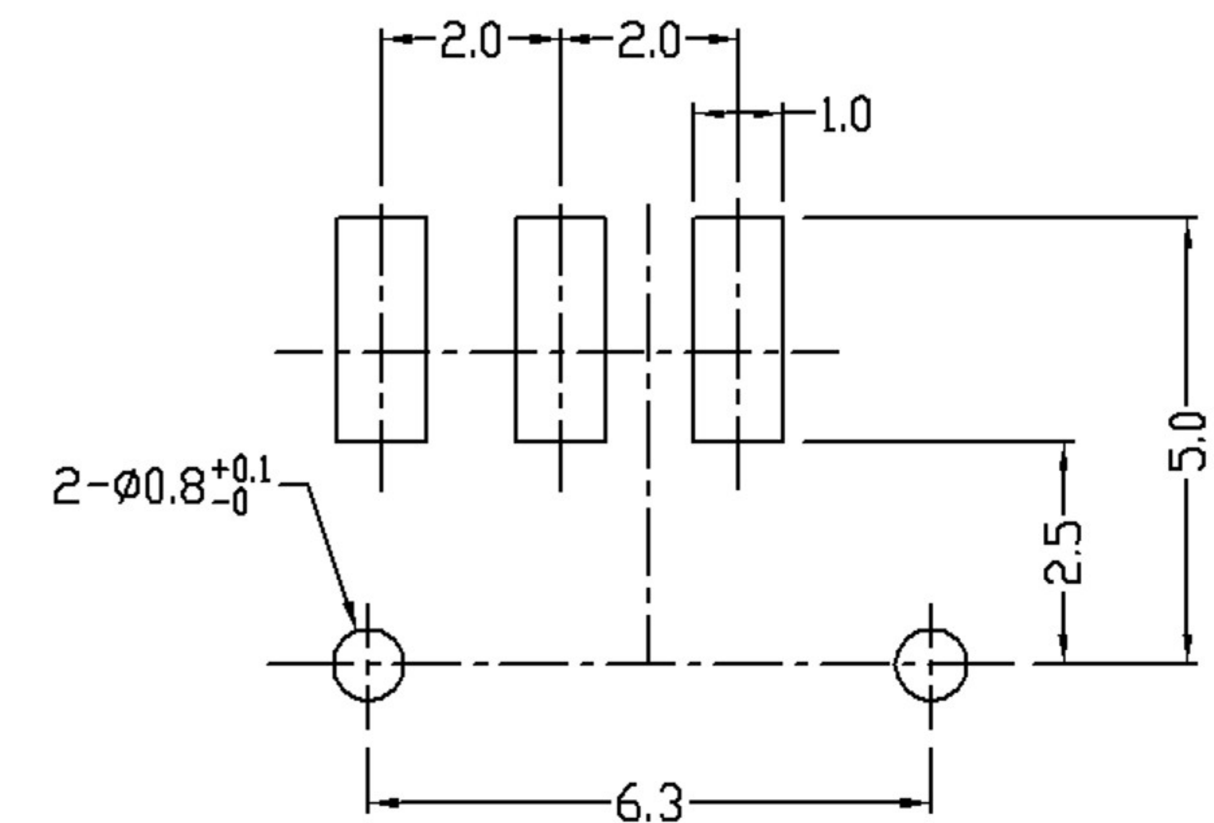
P.C.B. LAYOUT
