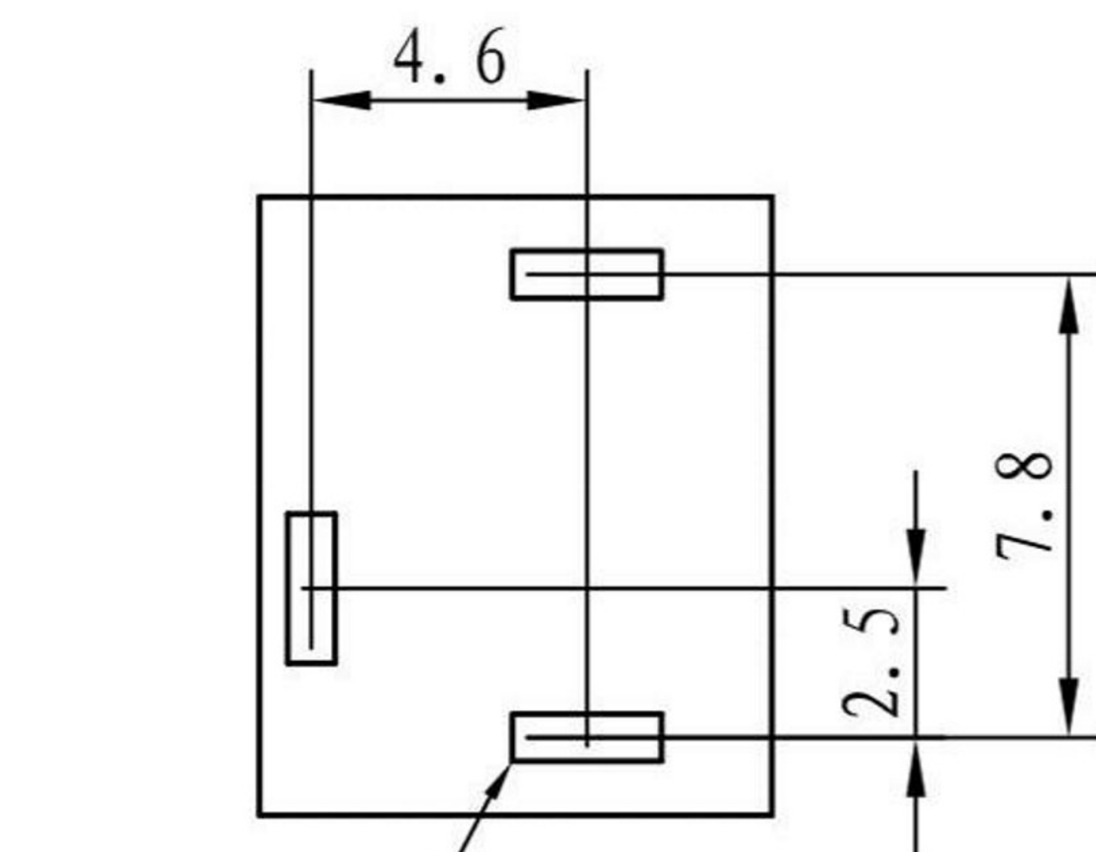
线路板安装尺寸示意图
