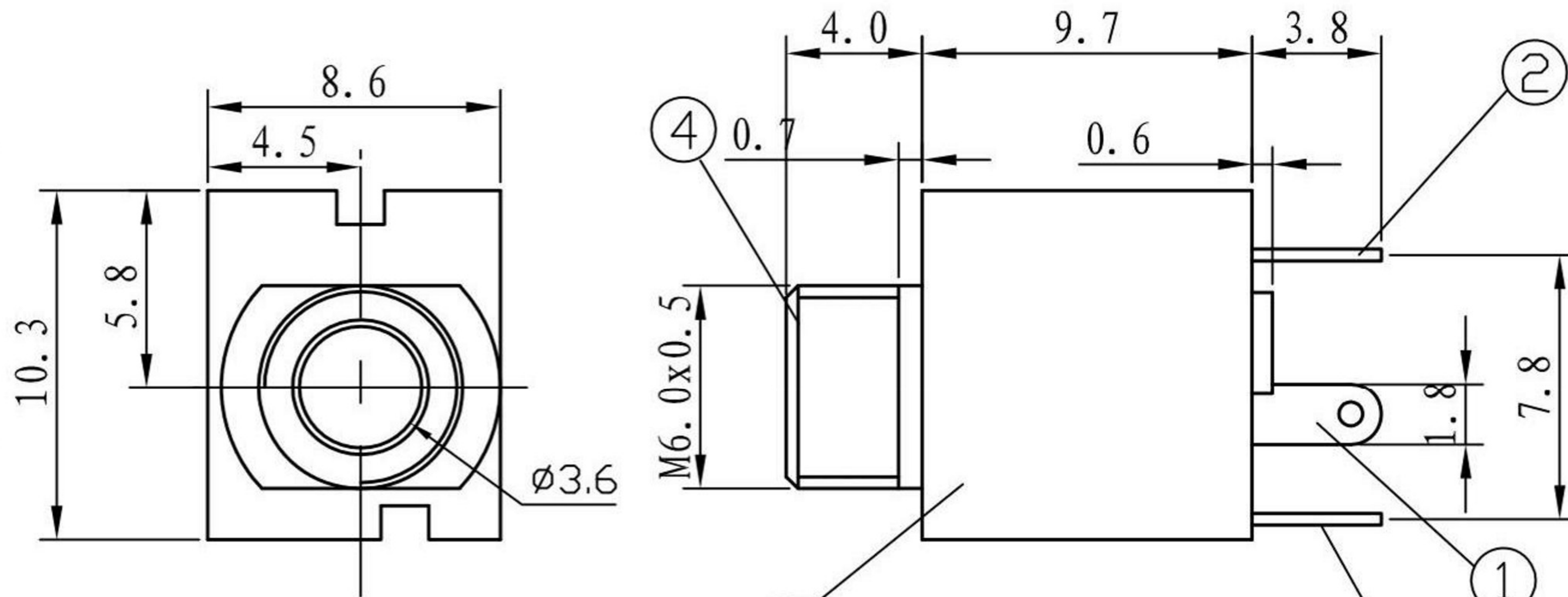
线路板安装尺寸示意图
