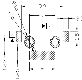
P.C.B LAND DIMENSION
