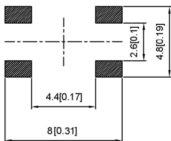
PCB Layout(pattern side)
