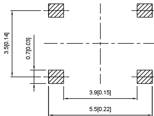
PCB LAYOUT(X0.5)
