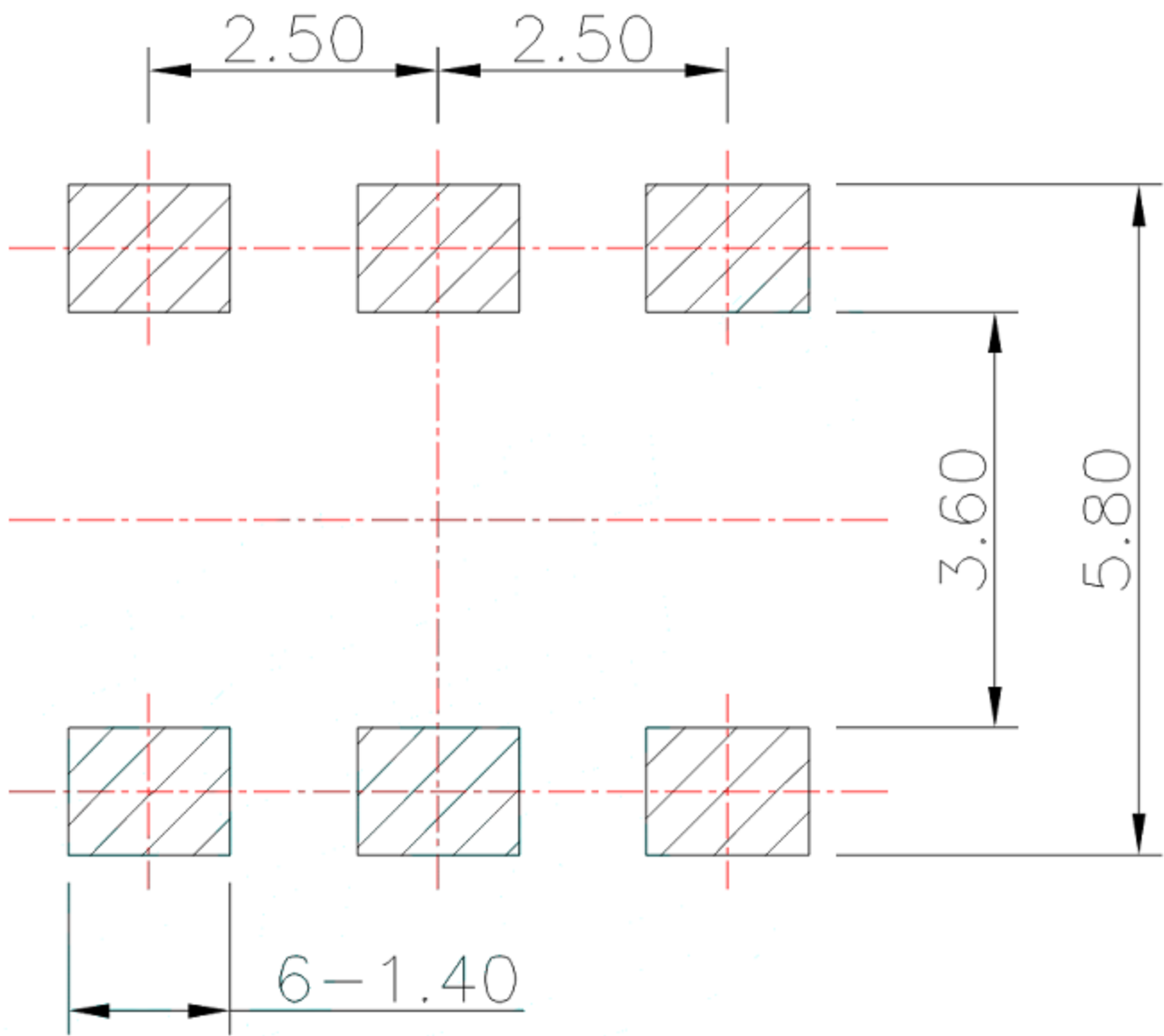
PCB Layout(Pattern side)
