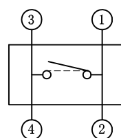
电路图：常开式(N.O) 1个电路1个接点 端子排列（自A方向看）
