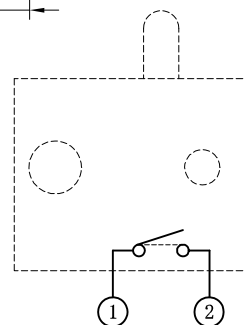
电路图：常开式 (N.O) 1个电路1个接点 端子排列 (自 A 方向看)
