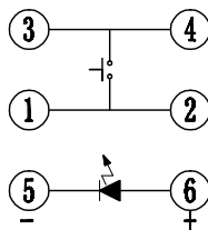
电原理图
