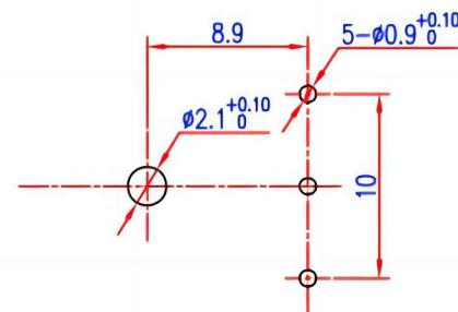
安装尺寸图
