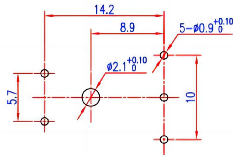
安装尺寸图
