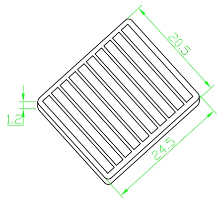
吸塑盒
