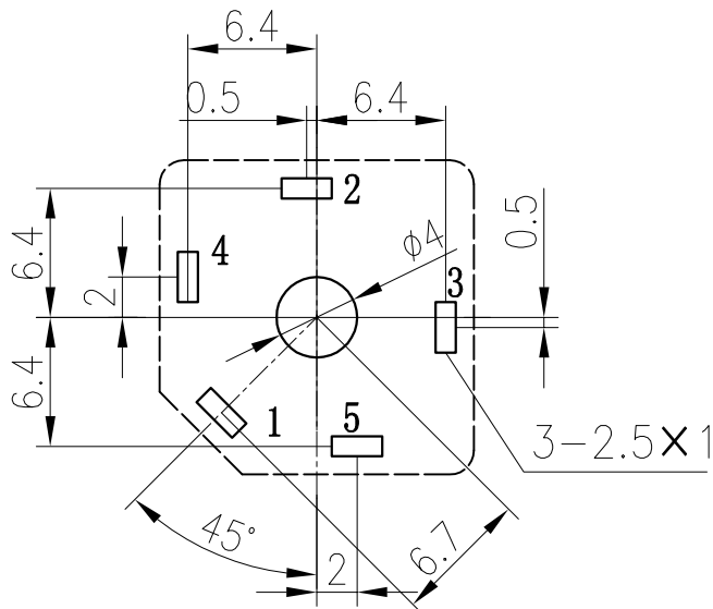
PCB尺寸图 TOP VIEW
