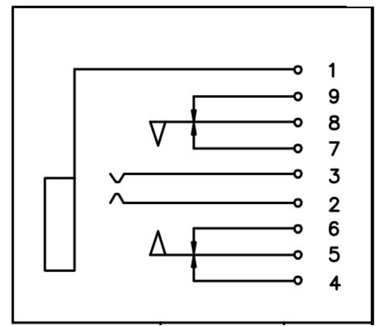
电路结构示意图
