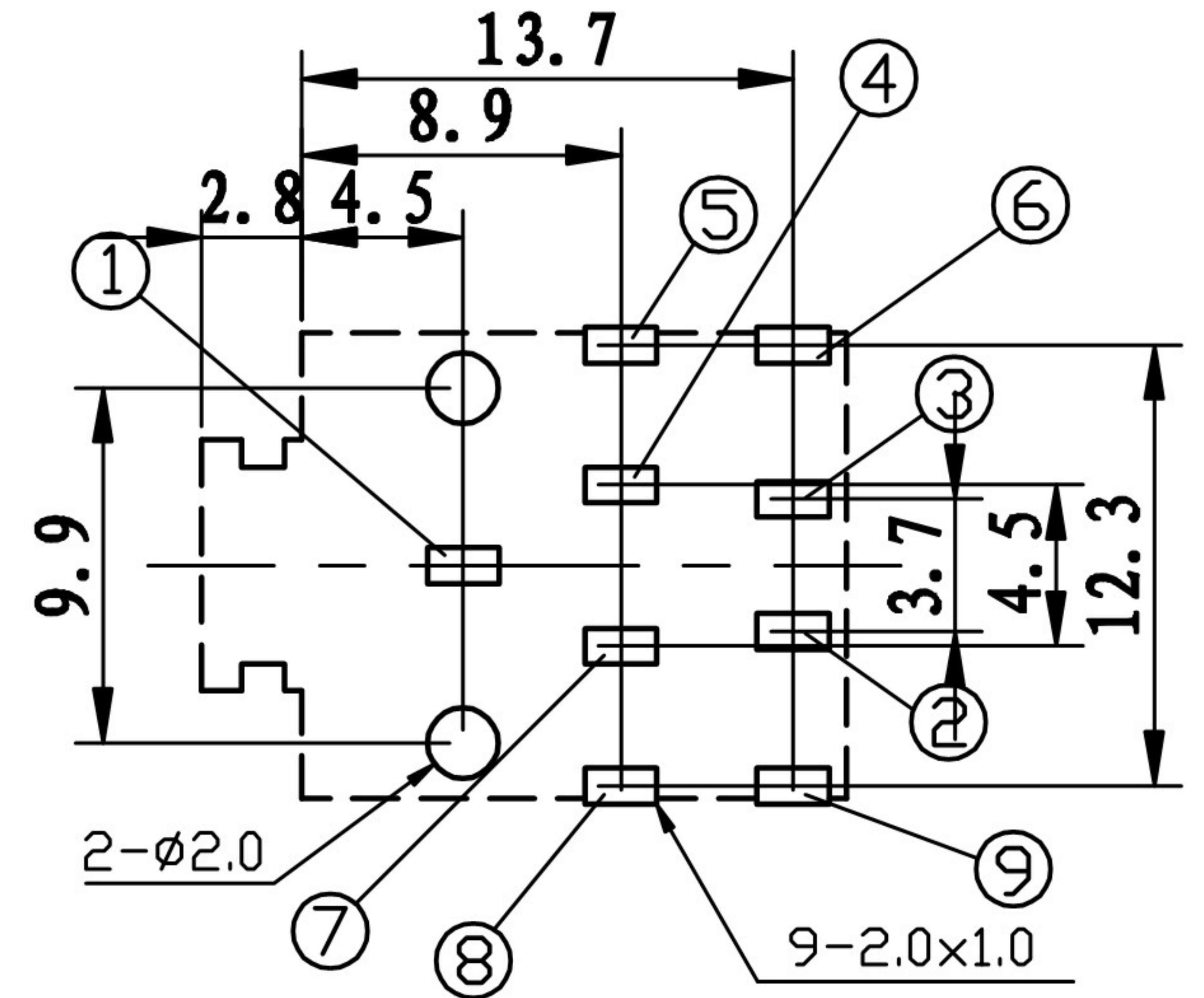
线路板安装尺寸示意图
