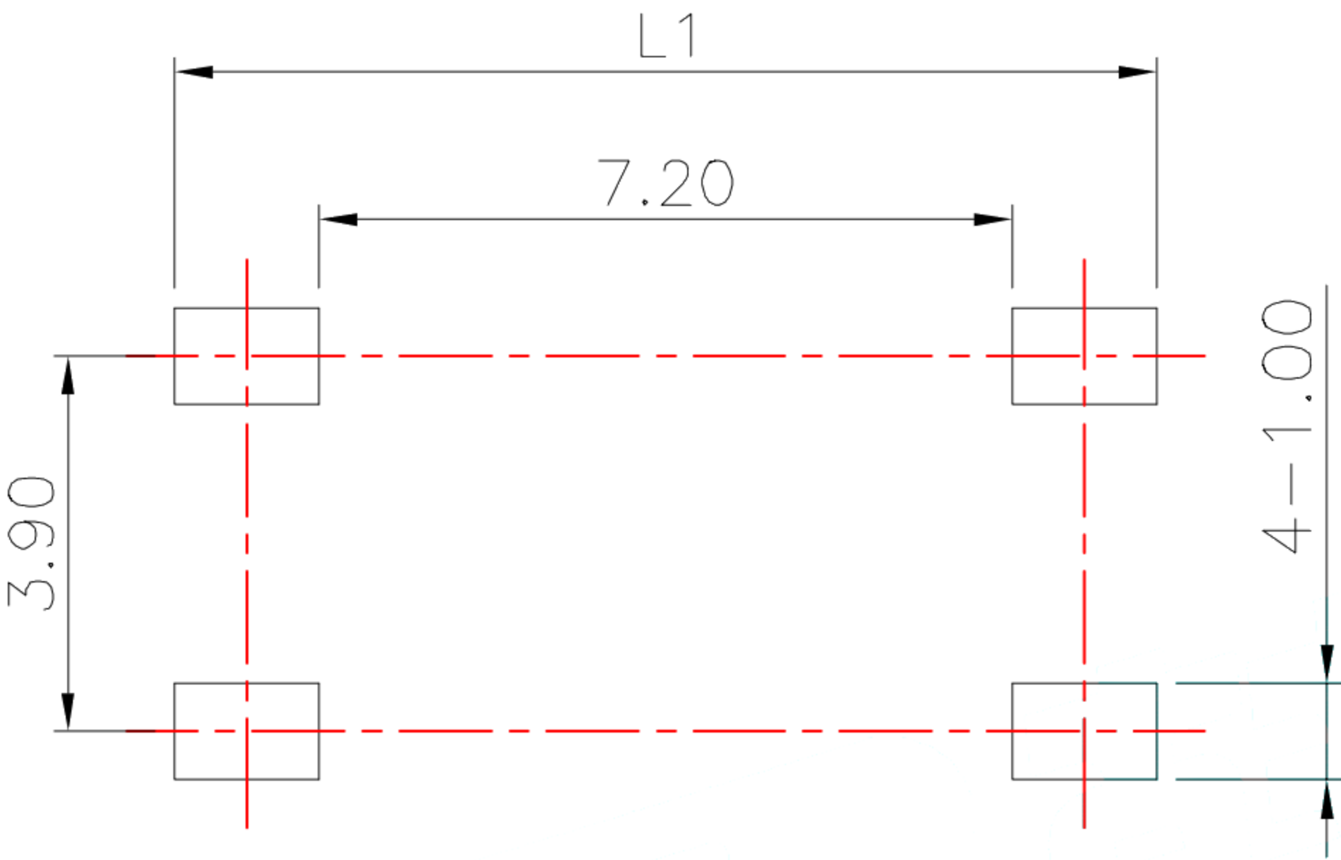
PCB Layout(Pattern side)
