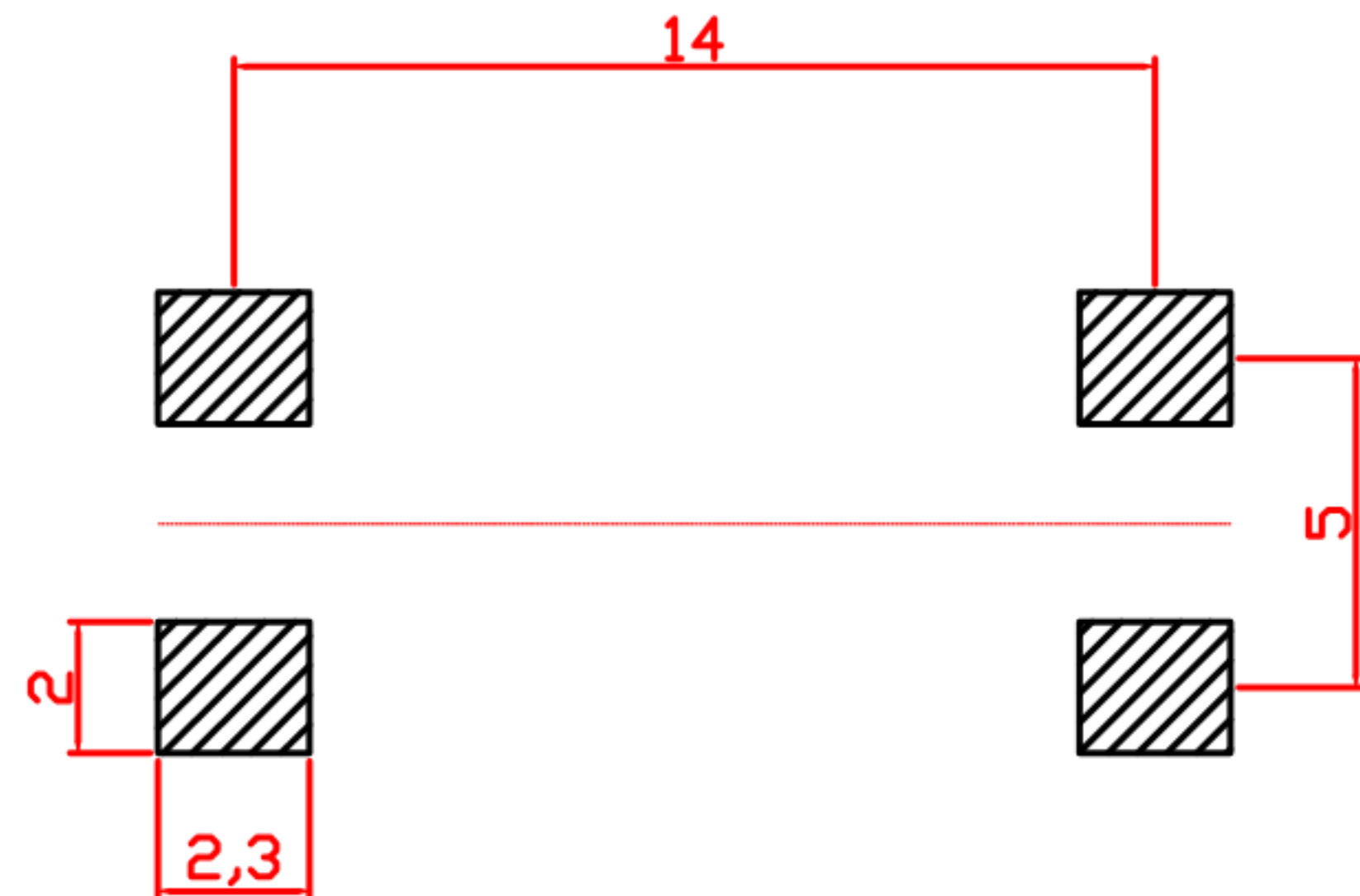
PCB焊接图
