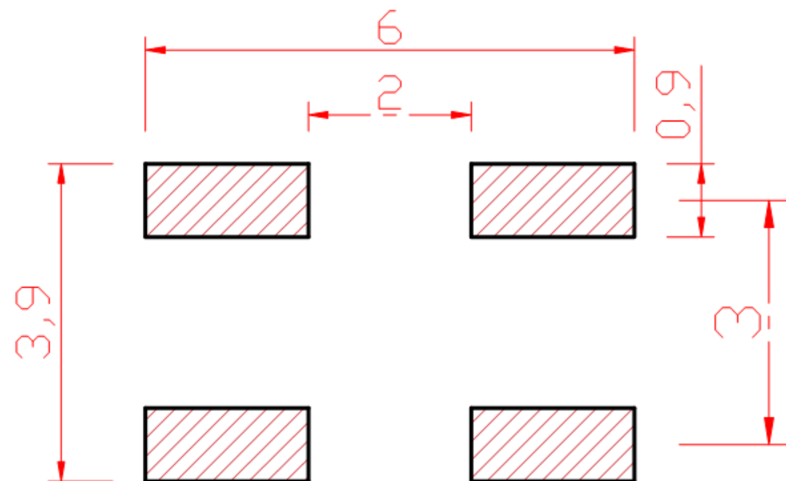
PCB. 焊接图
