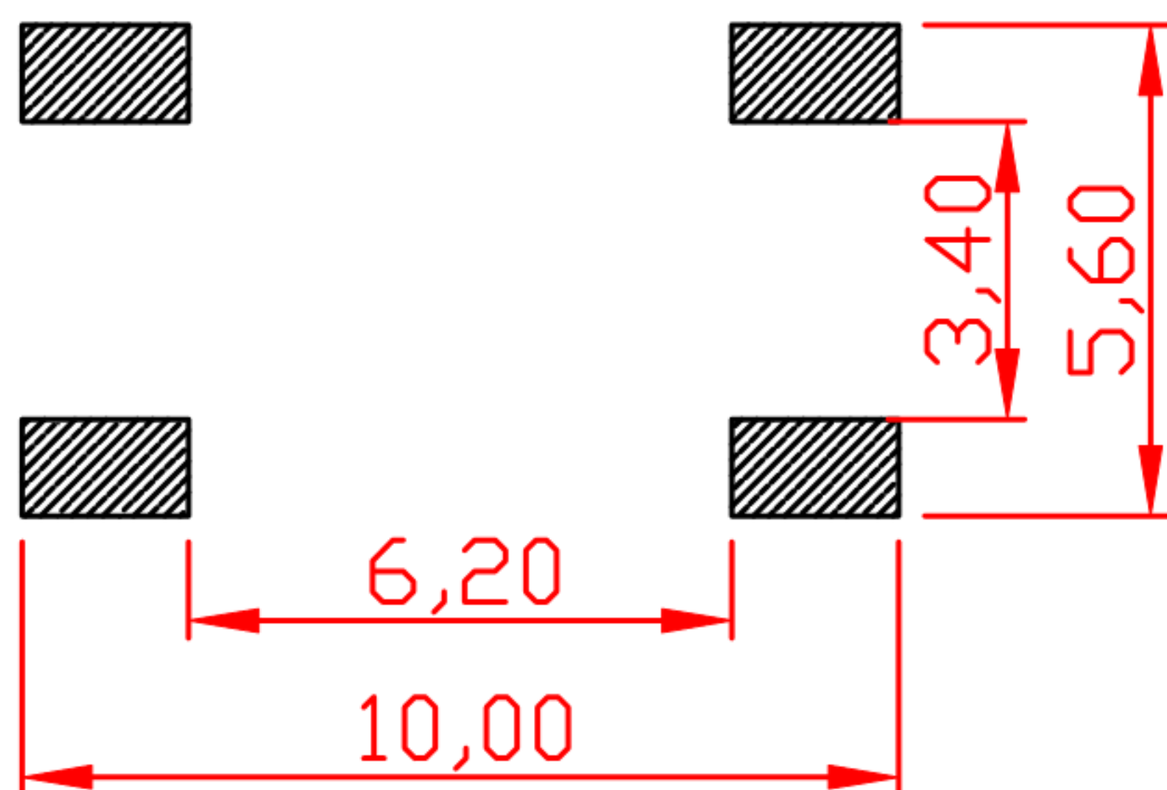
PCB. 焊接图
