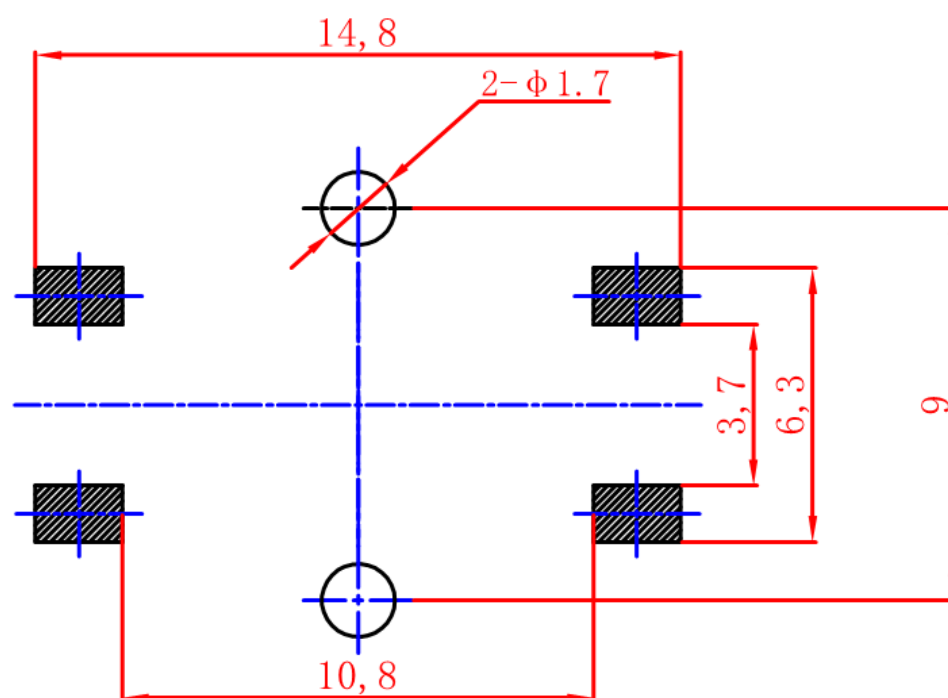
PCB. 焊接图
