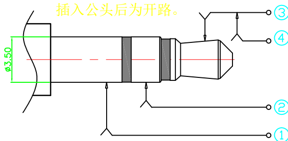
PULG SCHEMATIC
