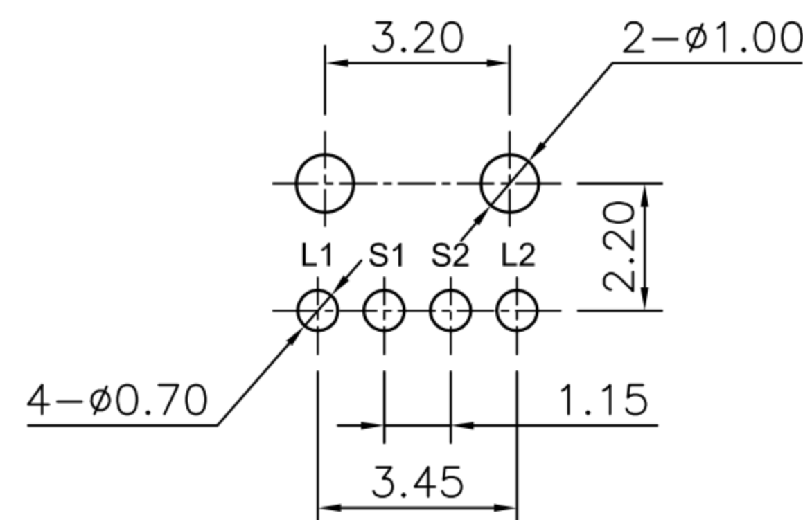
P.C.B.LAYOUT
