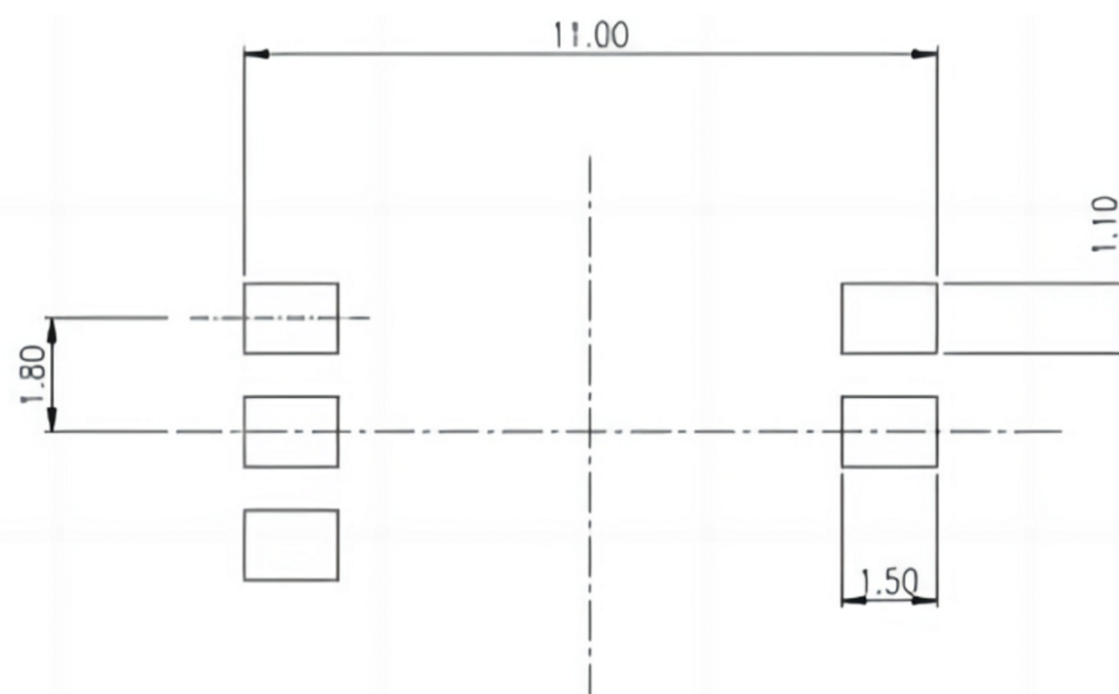
P.C.B. LAYOUT
