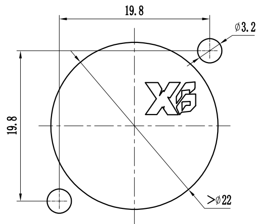
按装孔尺寸图
