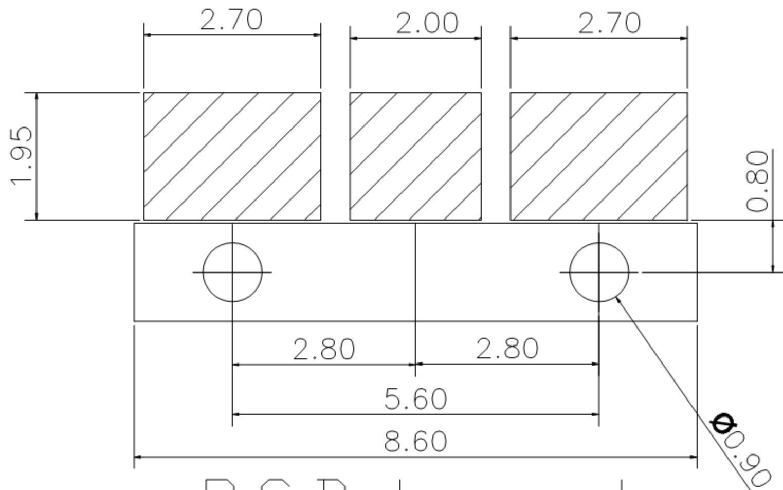
P.C.B Layout 图为焊盘位置和大小
