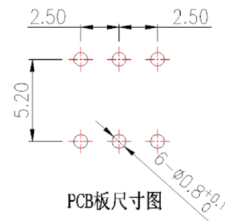
安装孔尺寸图
