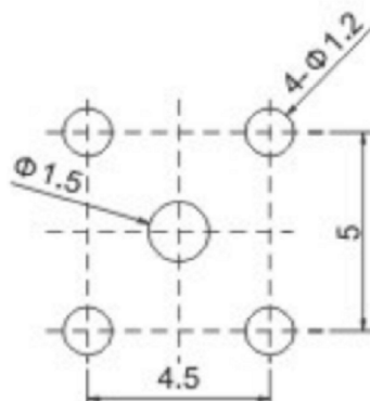
P.C.Board Dimension
