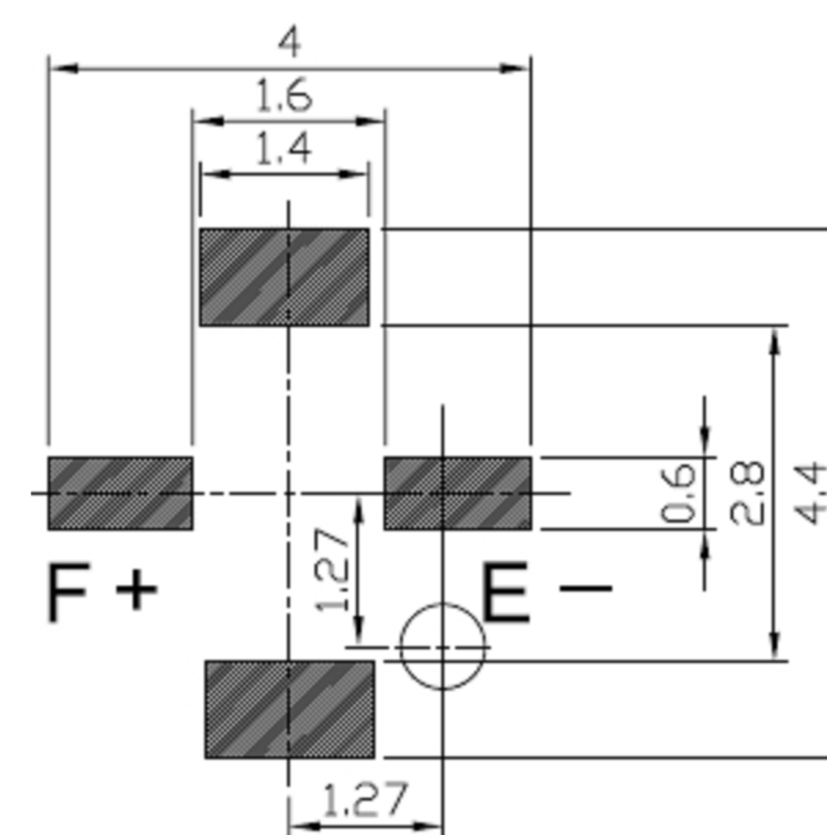
安装尺寸图
