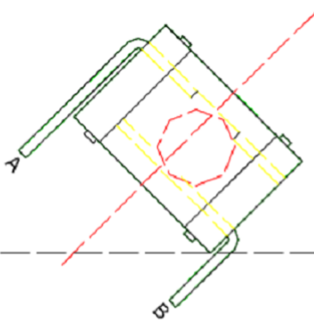
图二:顺时针方向旋转45° AB端子导通(ON)
