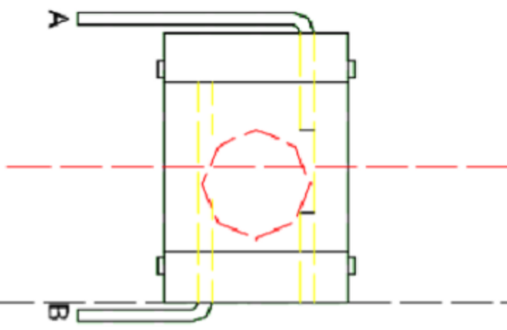
图三:顺时针方向旋转90° AB端子导通(ON)
