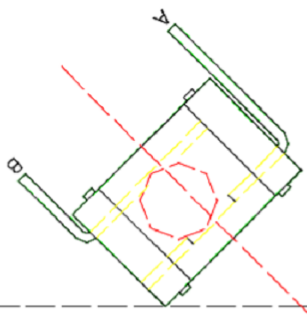
图四:顺时针方向旋转135° AB端子导通(ON)
