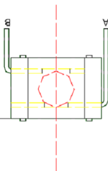
图五:顺时针方向旋转135° AB端子断开(OFF)
