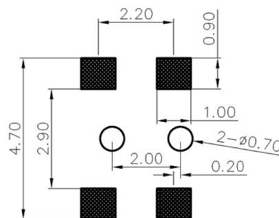
安装尺寸
