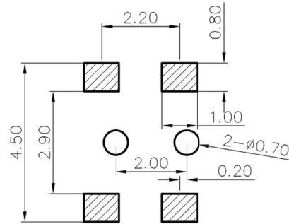
安装尺寸
