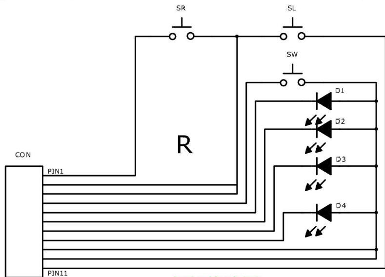
灯板线路图
