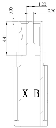
剖視圖
