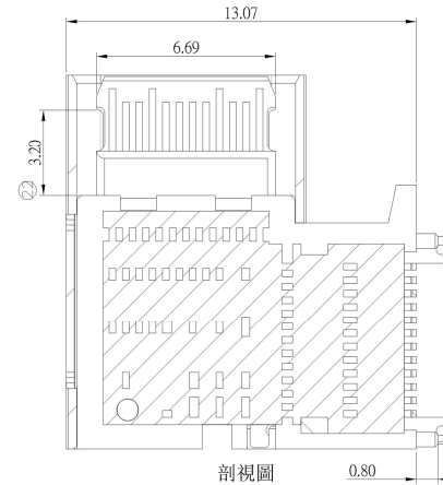
剖視圖
