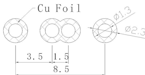
P. C. B. Layout (DIP) 焊盘位
