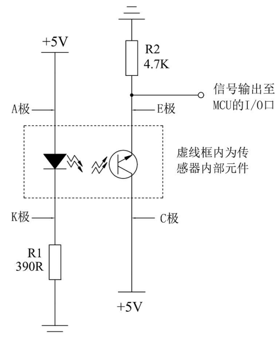
应用电路图
