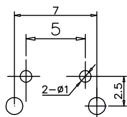
安装孔位图
